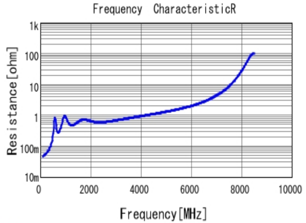
■ GRM1885C1H561JA01 R DCOV, 25degC
