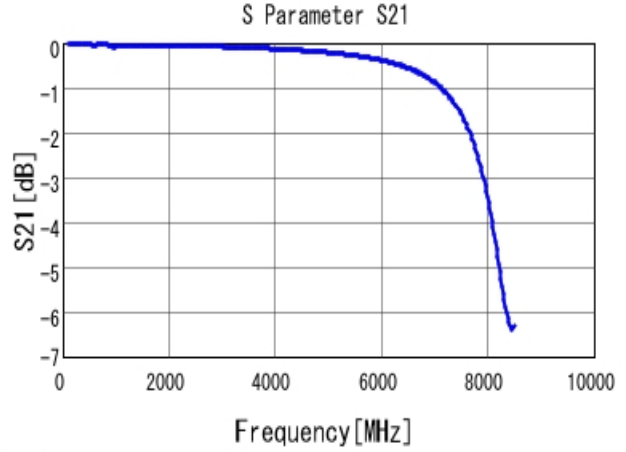
■ GRM1885C1H561JA01 S21 DCOV, 25degC
