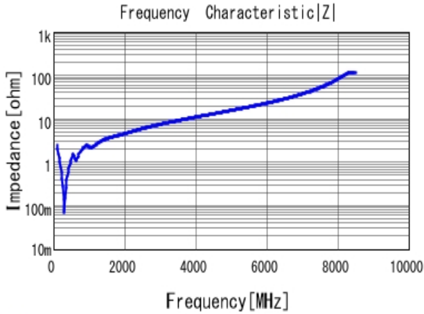
■ GRM1885C1H561JA01 |Z| DCOV, 25degC
