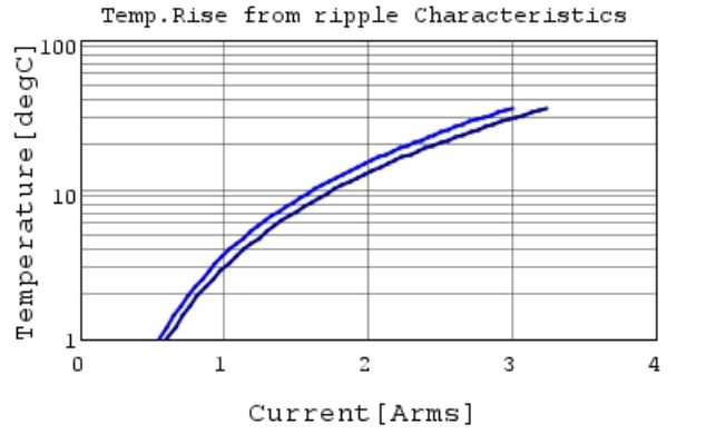
GRM033R60J225ME15 Temp.rise — 500kHz
