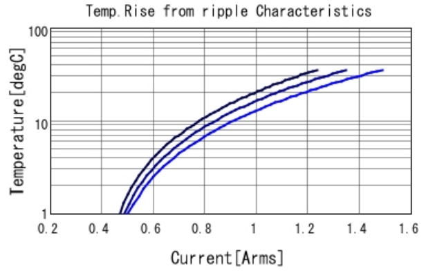
GJM1555C1H470JB01 Temp. rise — 500MHz — 700I
