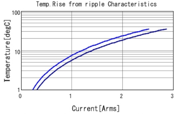
GCH188R71C105KE01 Temp. rise — 500kHz — 1MHz
