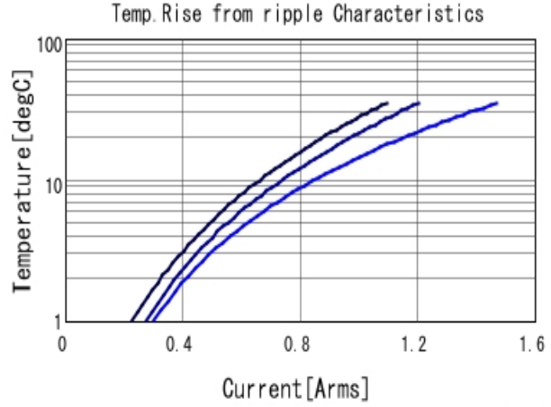
GRM1552C1E560JA01 Temp. rise ■ 200MHz ■ 500MHz ■ 700M
