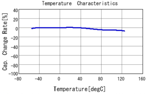
■ GCJ188R71H393KA12 C-Temp. capchange, DCO. 0V, AC1. 0Vrm
