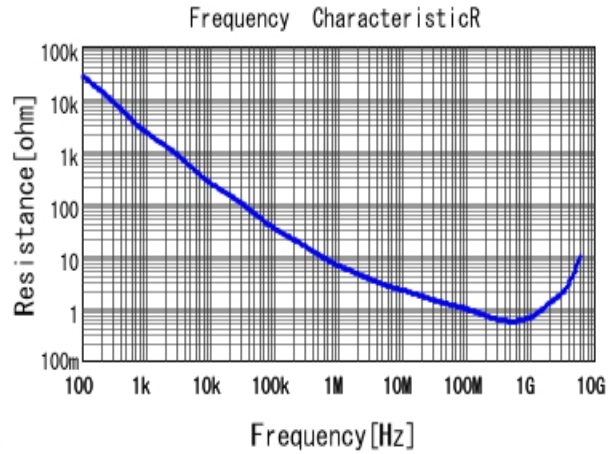
■ GRM155B11H331KA01 R DCOV, 20degC
