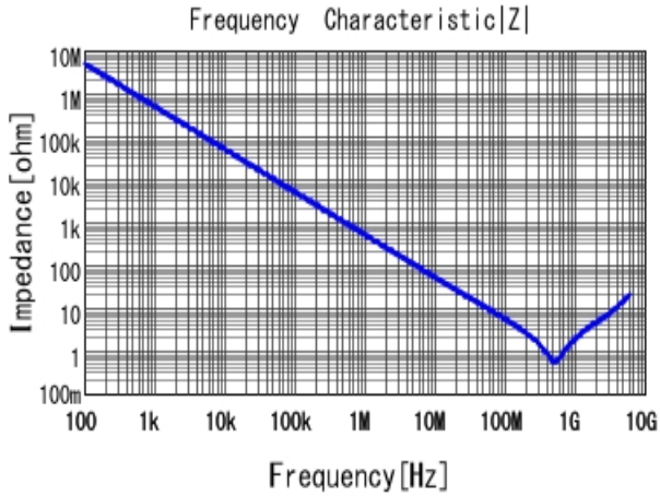
■ GRM155B11H331KA01 |Z| DCOV, 20degC
