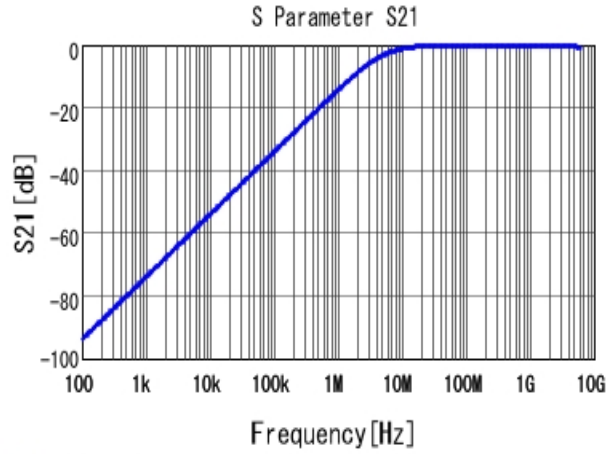
■ GRM155B11H331KA01 S21 DCOV, 20degC
