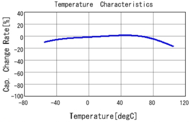
■ GRT155C80J475ME13 C-Temp. capchange, DCO. 0V, ACO. 1V rm
