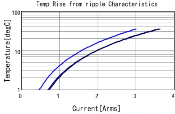
■ GRT155C80J475ME13 Temp. rise ■ 100kHz ■ 500kHz ■ 1MHz
