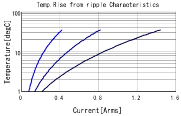
GC332DD72J333KX01 Temp. rise ■ 30kHz ■ 100kHz ■ 300kHz
