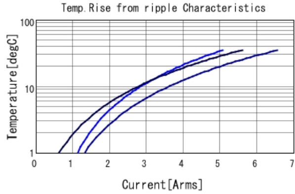
GRM32DC81E106KA12 Temp. rise — 80kHz — 400kHz
