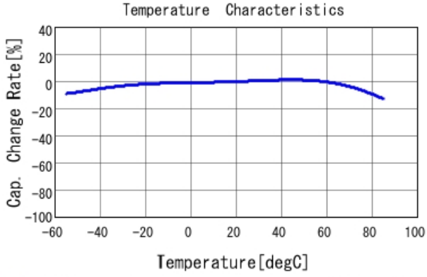
■ GRM188R60J226ME15 C-Temp. capchange, DCO. 0V, ACO. 2Vrm
