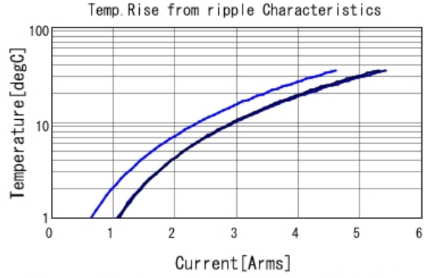
GRM188R60J226ME15 Temp. rise ■ 80kHz ■ 400kHz ■ 800kHz
