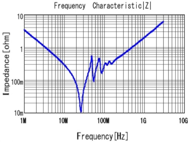
■ GRM32D7U2E473JW31 |Z| DCOV, 25degC
