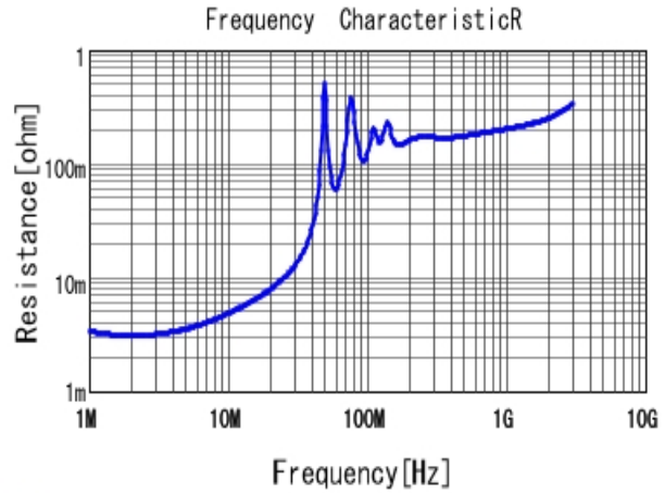
■ GRM32D7U2E473JW31 R DCOV, 25degC
