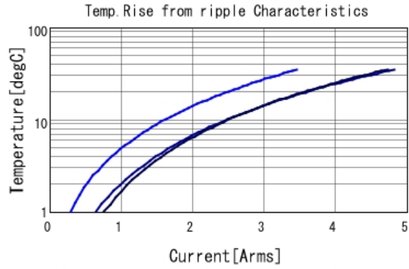
GRM319R6YA106MA12 Temp. rise — 80kHz — 400kHz
