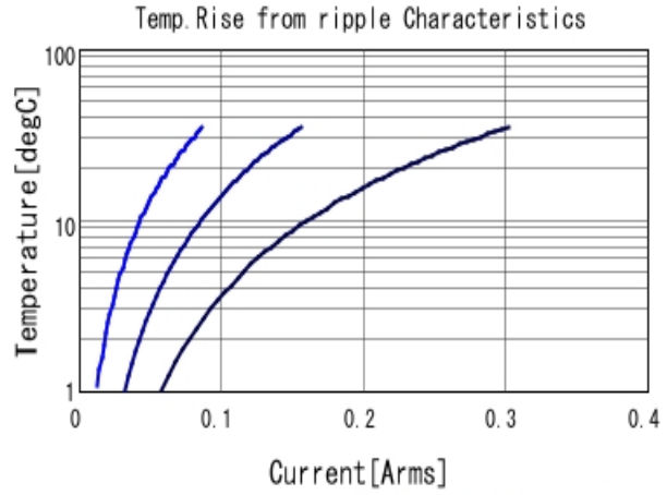
GRJ31BR72J472KWJ1 Temp. rise ■ 30kHz ■ 100kHz ■ 300kHz
