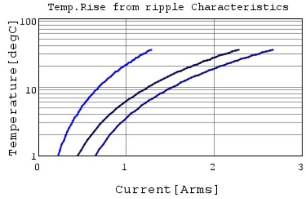
GCM21BR71H474KA55 Temp.rise — 100kHz —
