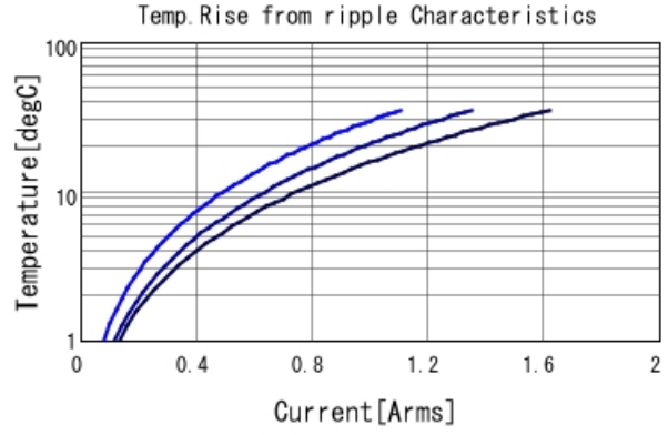
GRM155R61E224KE01 Temp. rise — 300kHz — 600I
