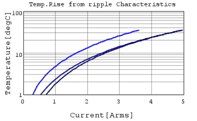
GRT188C81C106ME13 Temp.rise — 80kHz —
