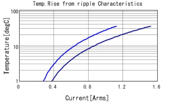
GRM155R60J104KA01 Temp. rise — 500kHz — 1MHz
