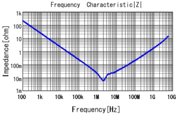
■ GCJ21BC71C106KE02 |Z| DC0V, 25degC
