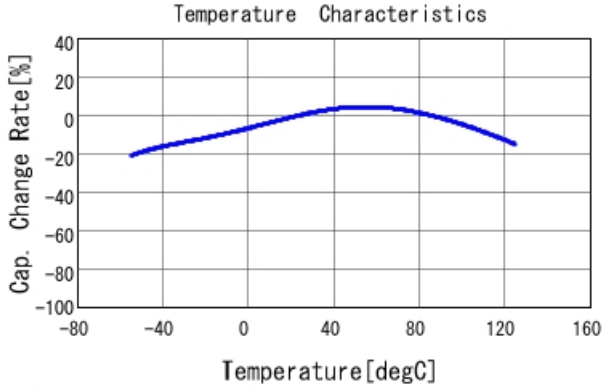
■ GCJ21BC71C106KE02 C-Temp. capchange, DCO. 0V, ACO. 2Vrm
