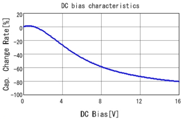
■ GCJ21BC71C106KE02 C-DC bias capchange, 25.0degC, AC1V
