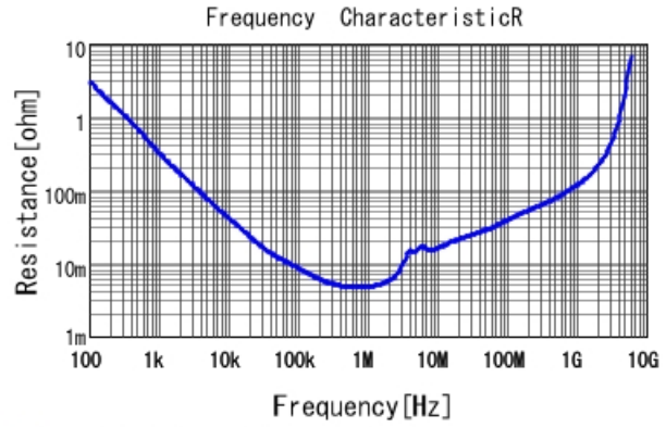
■ GCJ21BC71C106KE02 R DC0V, 25degC
