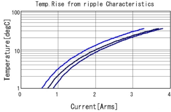
GCJ21BC71C106KE02 Temp. rise ■ 80kHz ■ 400kHz ■ 800kHz
