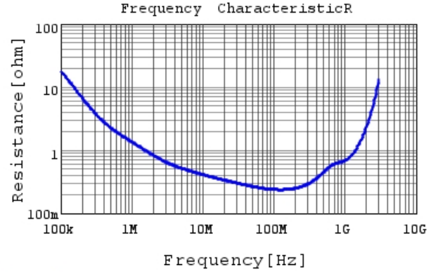
GCJ31BR73A222KXJ1 R DCOV, 25degC
