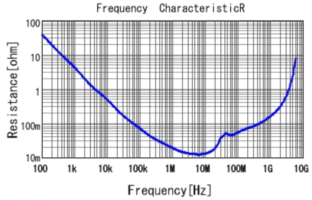
GRM188B31E224KA87 R DCOV, 20degC
