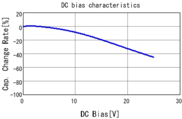
GRM188B31E224KA87 C-DC bias capchange, 20.0degC, A
