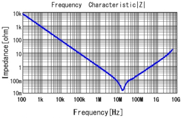
GRM188B31E224KA87 |Z| DCOV, 20degC
