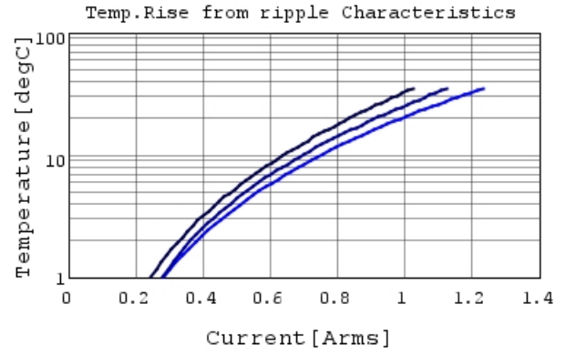
GRT1555C2A470JA02 Temp.rise 500MHz
