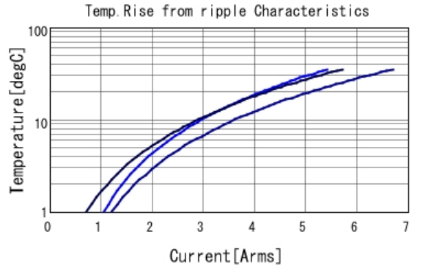
GRM32DR61C106KA01 Temp. rise — 80kHz — 400kHz
