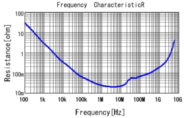
GCJ188R71C334KA01 R DCOV, 25degC
