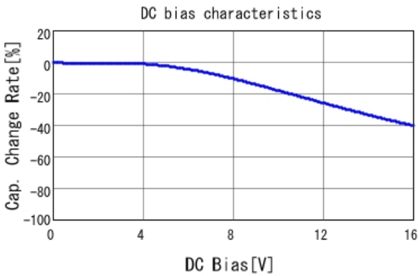
GCJ188R71C334KA01 C-DC bias capchange, 25.0degC, A
