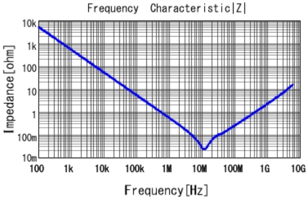
GCJ188R71C334KA01 |Z| DCOV, 25degC
