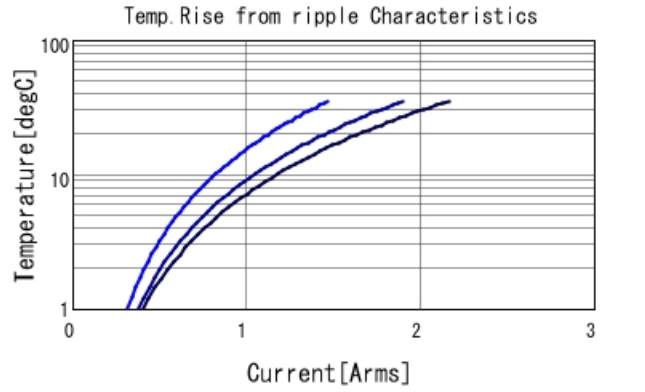
GCJ188R71C334KA01 Temp. rise — 300kHz — 600
