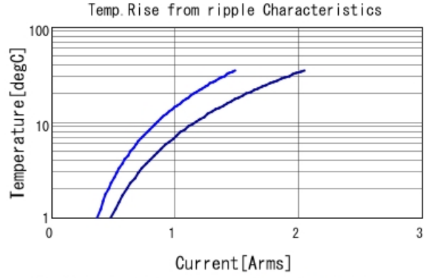
■ GCD21BR71H104MA01 Temp. rise ■ 500kHz ■ 1MHz
