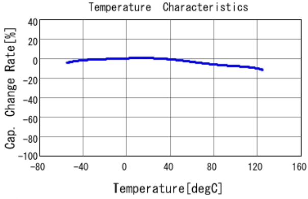
■ GCD21BR71H104MA01 C-Temp. capchange, DCO. 0V, AC1. 0Vrm
