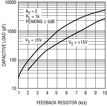
LT1217 • TPC10
