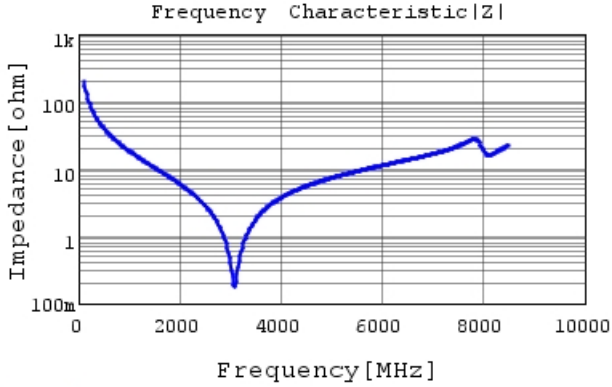
GCQ1555C1H7R8DB01 |Z| DC0V, 25degC
