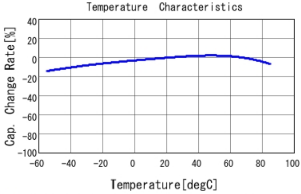
■ GRM033R61A393ME84 C-Temp. capchange, DCO. 0V, ACO. 5Vrm
