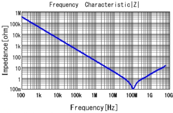
■ GCD188R72A472MA01 |Z| DCOV, 25degC
