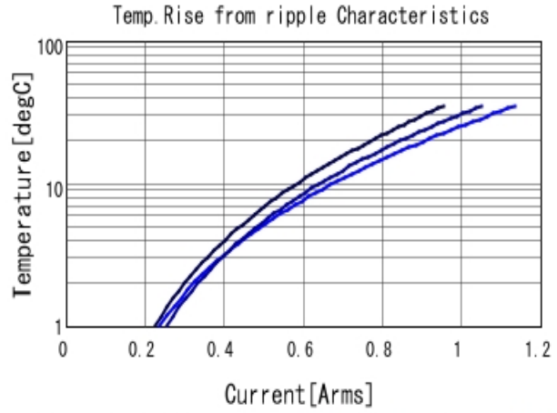
GRM1552C1H330JA01 Temp. rise ■ 500MHz ■ 700MHz ■ 1GHz
