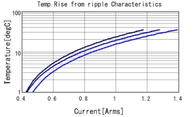
GJM1555C1H330FB01 Temp. rise — 500MHz — 700I
