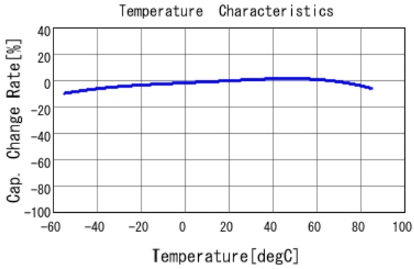
■ GRT155R61A475ME13 C-Temp. capchange, DCO. 0V, ACO. 1V rm
