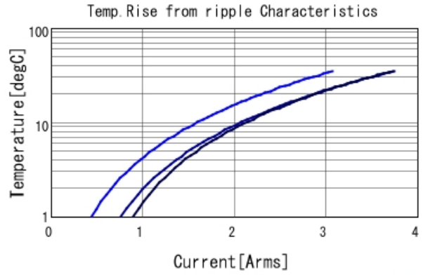
■ GRT155R61A475ME13 Temp. rise ■ 100kHz ■ 500kHz ■ 1MHz
