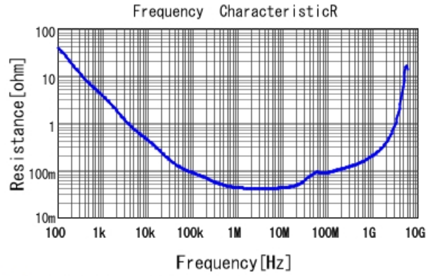
■ GCJ188R71H154KA01 R DCOV, 25degC
