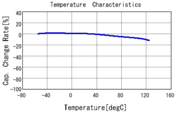
■ GCJ188R71H154KA01 C-Temp. capchange, DCO. 0V, AC1. 0Vrm
