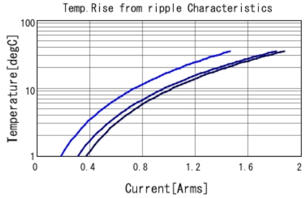
GCJ188R71H154KA01 Temp. rise ■ 400kHz ■ 800kHz ■ 1MHz
