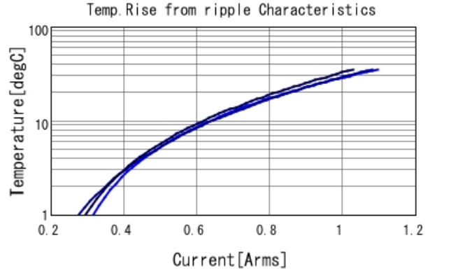
GQM2195G2E5R1DB12 Temp. rise — 700MHz — 1GHz
