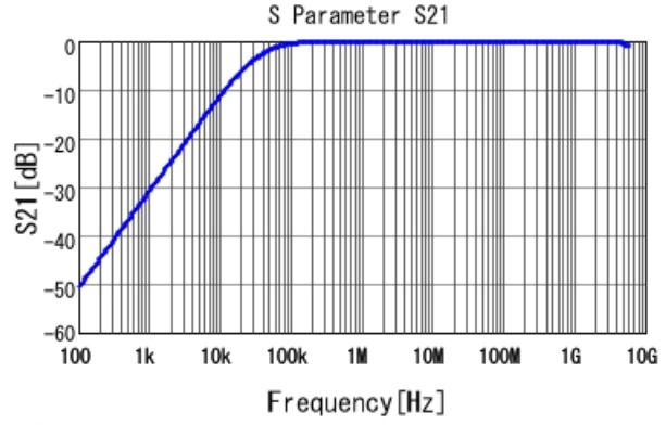
■ GCD21BR71H473MA01 S21 DCOV, 25degC
