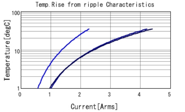
GCM32ER71H105KA37 Temp. rise — 100kHz — 500
