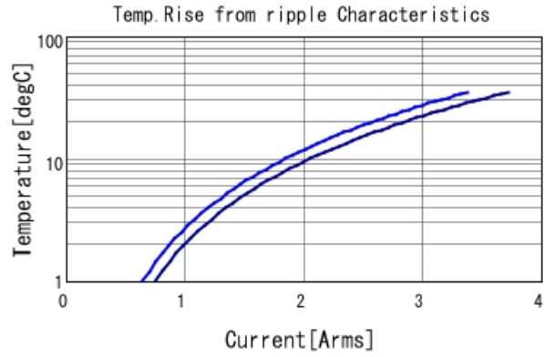
■ GRT155C81C225KE13 Temp. rise ■ 500kHz ■ 1MHz
