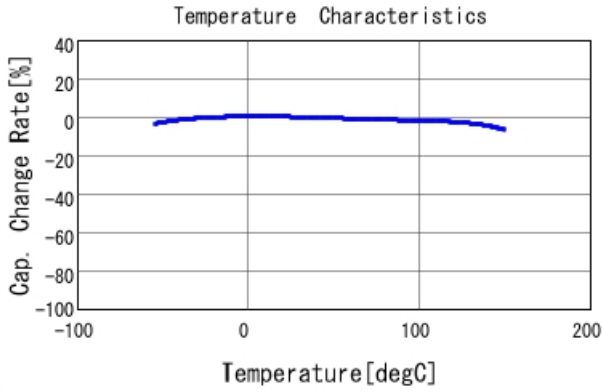
■ GCJ188R92A683KA01 C-Temp. capchange, DCO. 0V, AC1. 0Vrm
