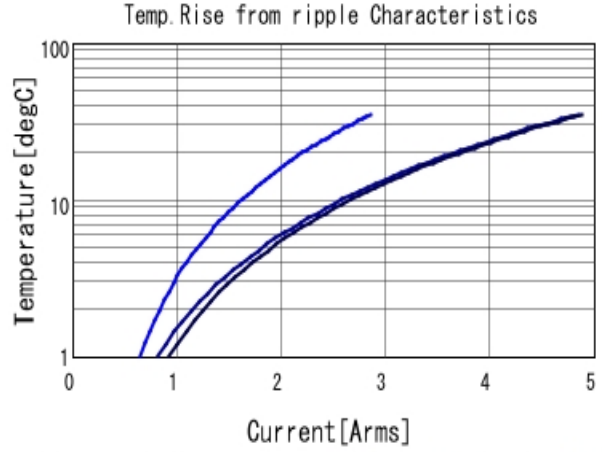
GRM31MR11C225KA35 Temp. rise ■ 100kHz ■ 500kHz ■ 1MHz
