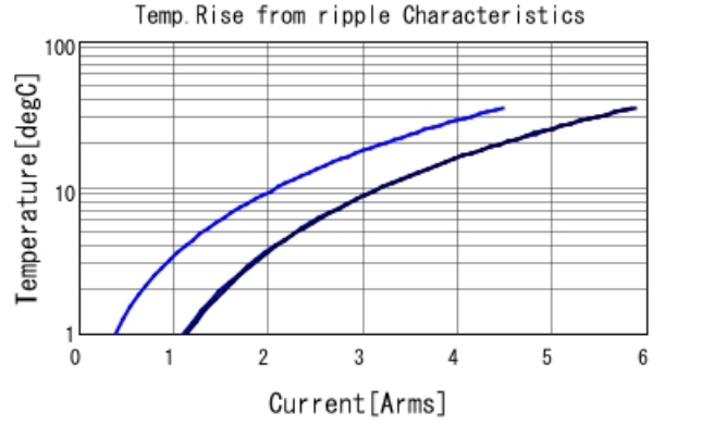
GRM319R61A226ME15 Temp. rise — 80kHz — 400kHz
