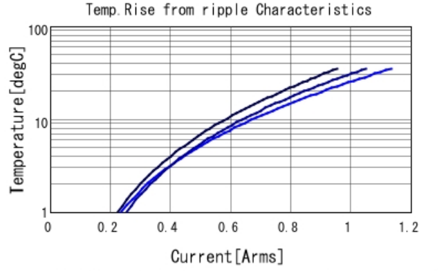
GRM1555C1E330JA01 Temp. rise — 500MHz — 700I
