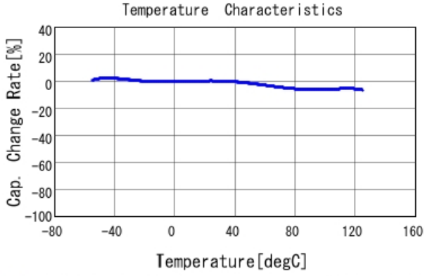
■ GCJ188R71H682KA01 C-Temp. capchange, DCO. 0V, AC1. 0Vrm
