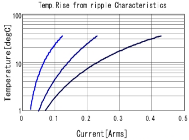
GRJ32QR73A103KWJ1 Temp. rise ■ 30kHz ■ 100kHz ■ 300kHz
