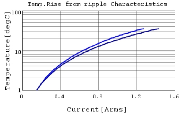
GRM033R61E224KE01 Temp.rise — 600kHz
