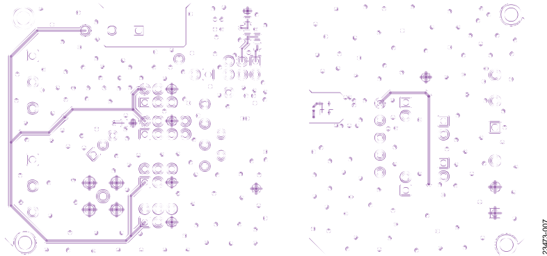
Figure 10. EVAL-ADM2563EEBZ/EVAL-ADM2863EEBZ, Layer 2
