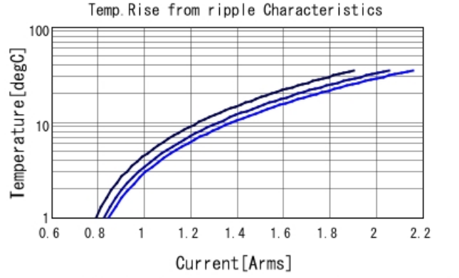
GQM1555C2D150JB01 Temp. rise — 500MHz — 700I
