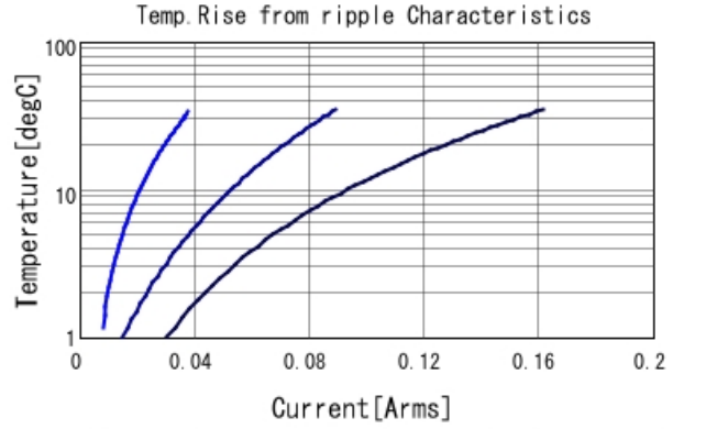
GRM31AR72J222KW01 Temp. rise — 30kHz — 100kHz
