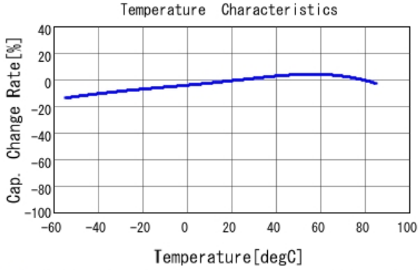
■ GRM033R60J273KE01 C-Temp. capchange, DCO. 0V, ACO. 5Vrm
