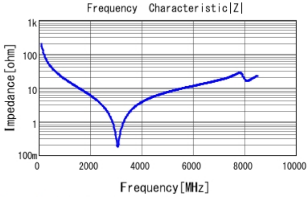
GCQ1555C1H7R8CB01 |Z| DC0V, 25degC
