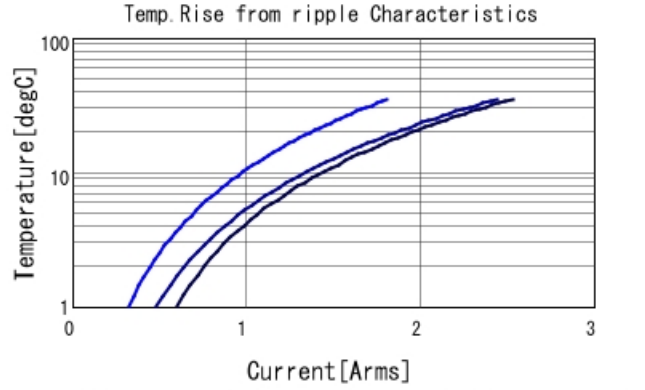
GRM219R71H334KA88 Temp. rise — 300kHz — 600I
